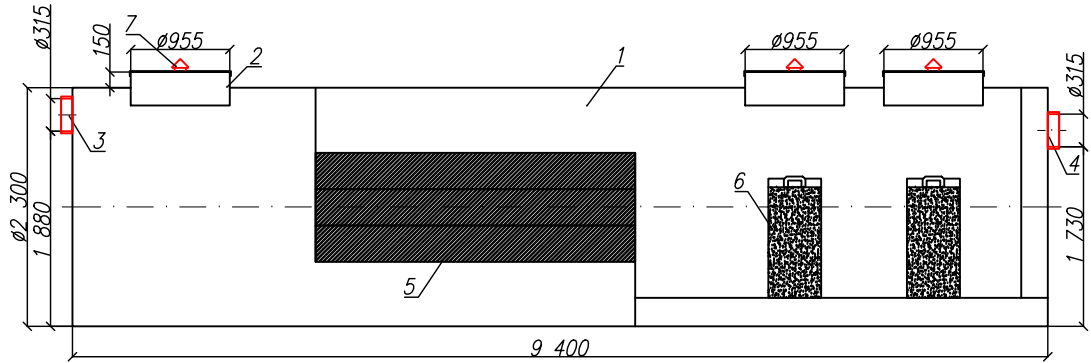
Разрез 1-1
