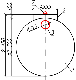
Вид спереди
