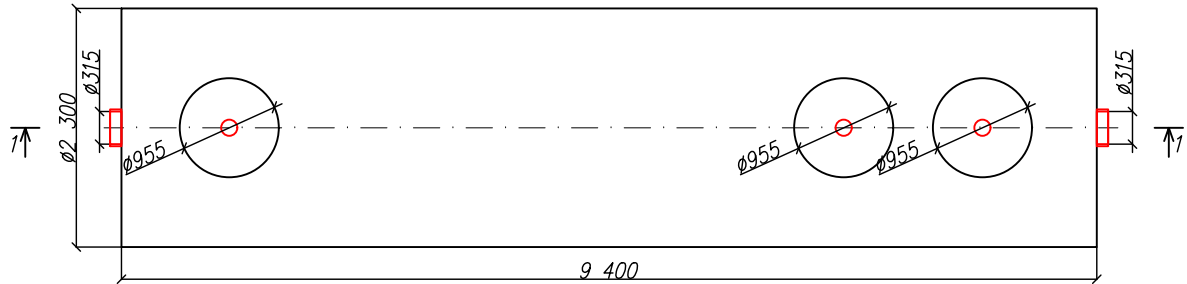
Вид сверху
