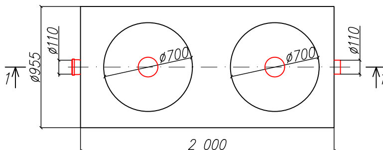
Вид сверху
