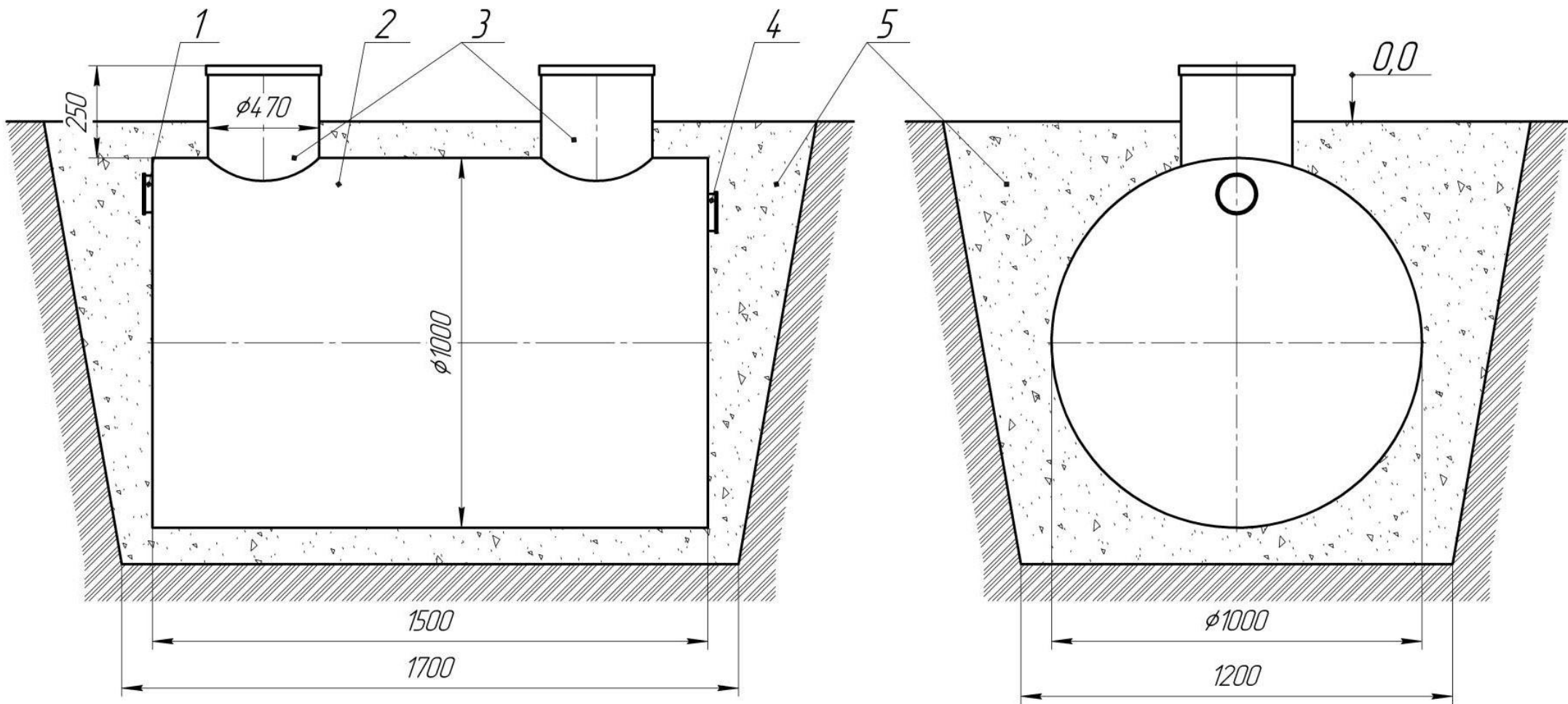
Рисунок А.1 Монтаж Энергонезависимого септика «Дрена-БИО 3» на подготовленное песчаное основание
