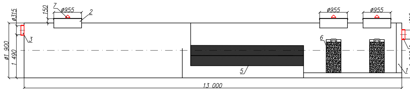
Разрез 1-1
