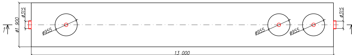
Вид сверху
