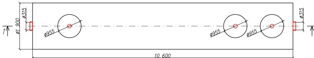
Вид сверху
