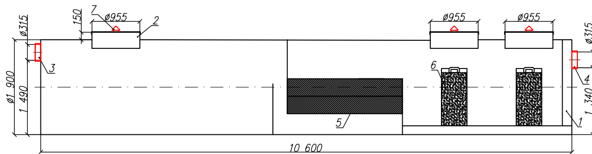
Разрез 1-1
