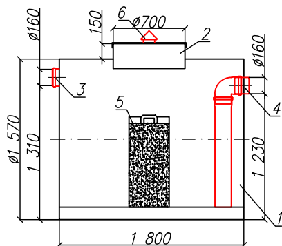
Разрез 1-1
