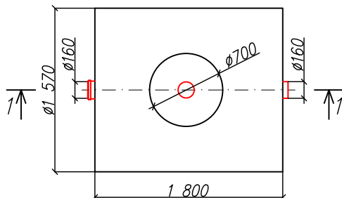
Вид сверху
