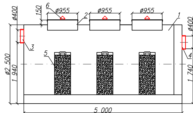
Разрез 1-1
