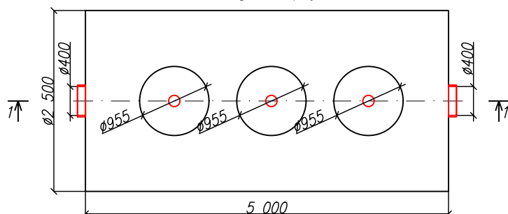
Вид сверху
