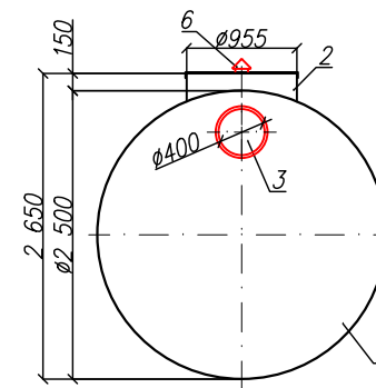
Вид спереди
