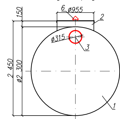
Вид спереди
