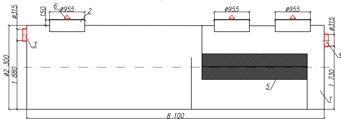
Вид сверху
