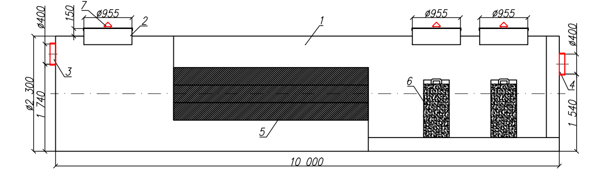
Разрез 1-1
