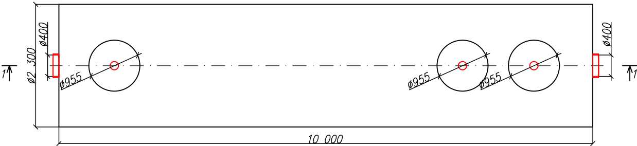
Вид сверху
