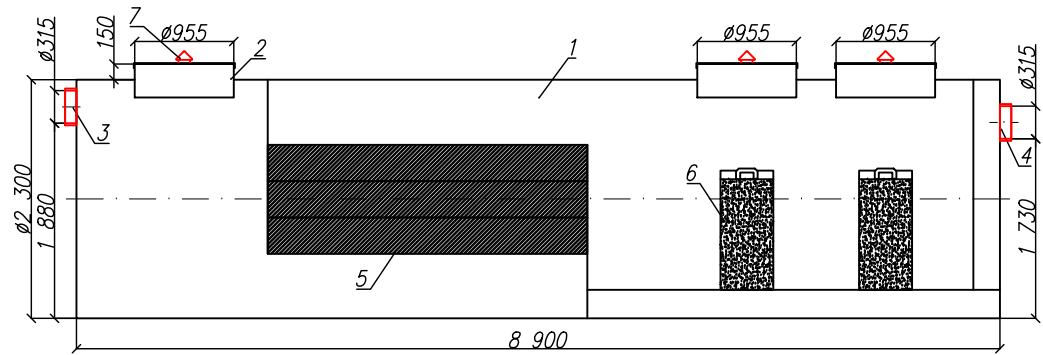
Разрез 1-1
