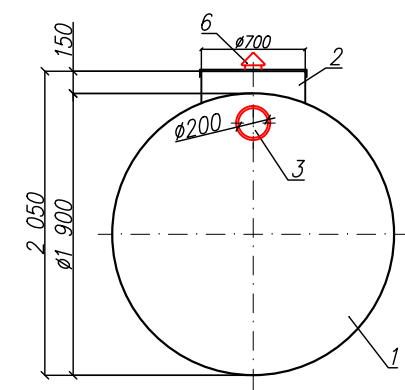
Вид спереди
