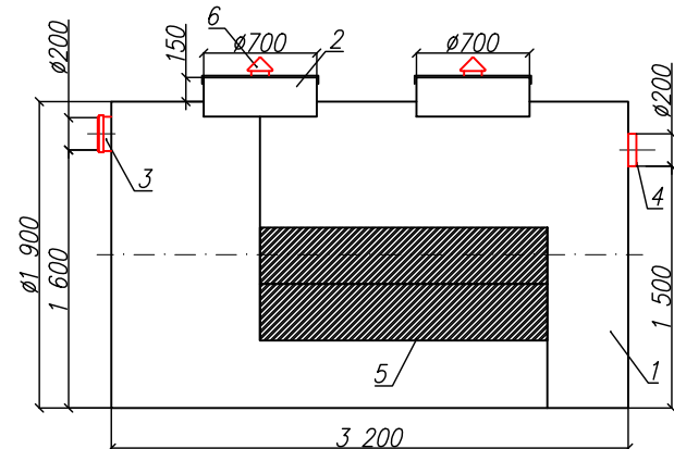
Разрез 1-1
