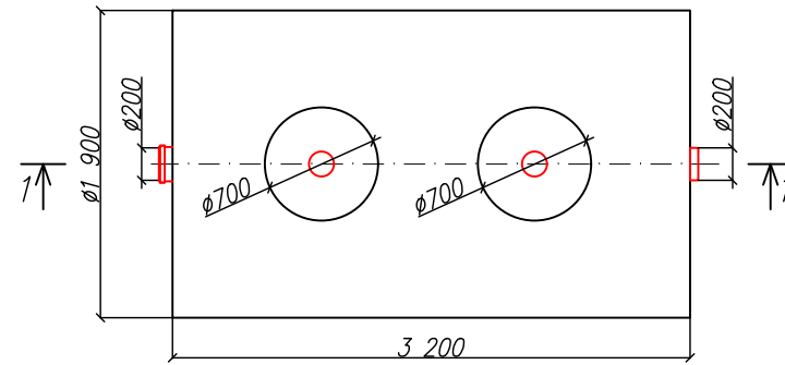
Вид сверху
