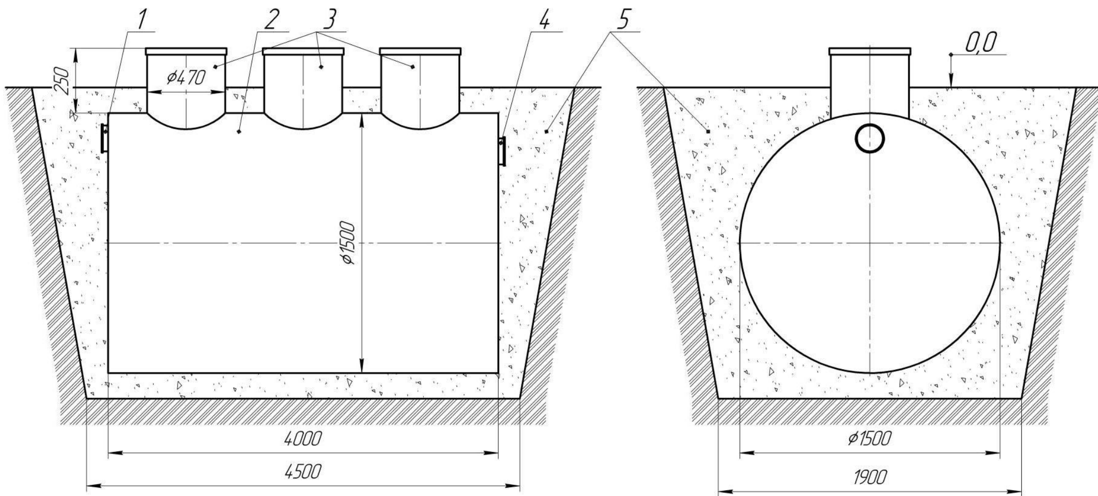
Рисунок А.1 Монтаж жироуловителя «Жирожор 72-4800» на подготовленное песчаное основание
