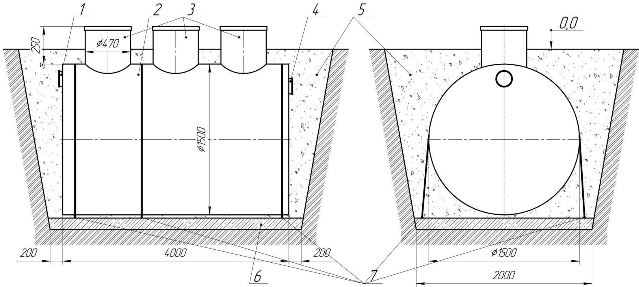
Рисунок А.1 Монтаж жироуловителя «Жирожор 72-4800» на ж/б основание
