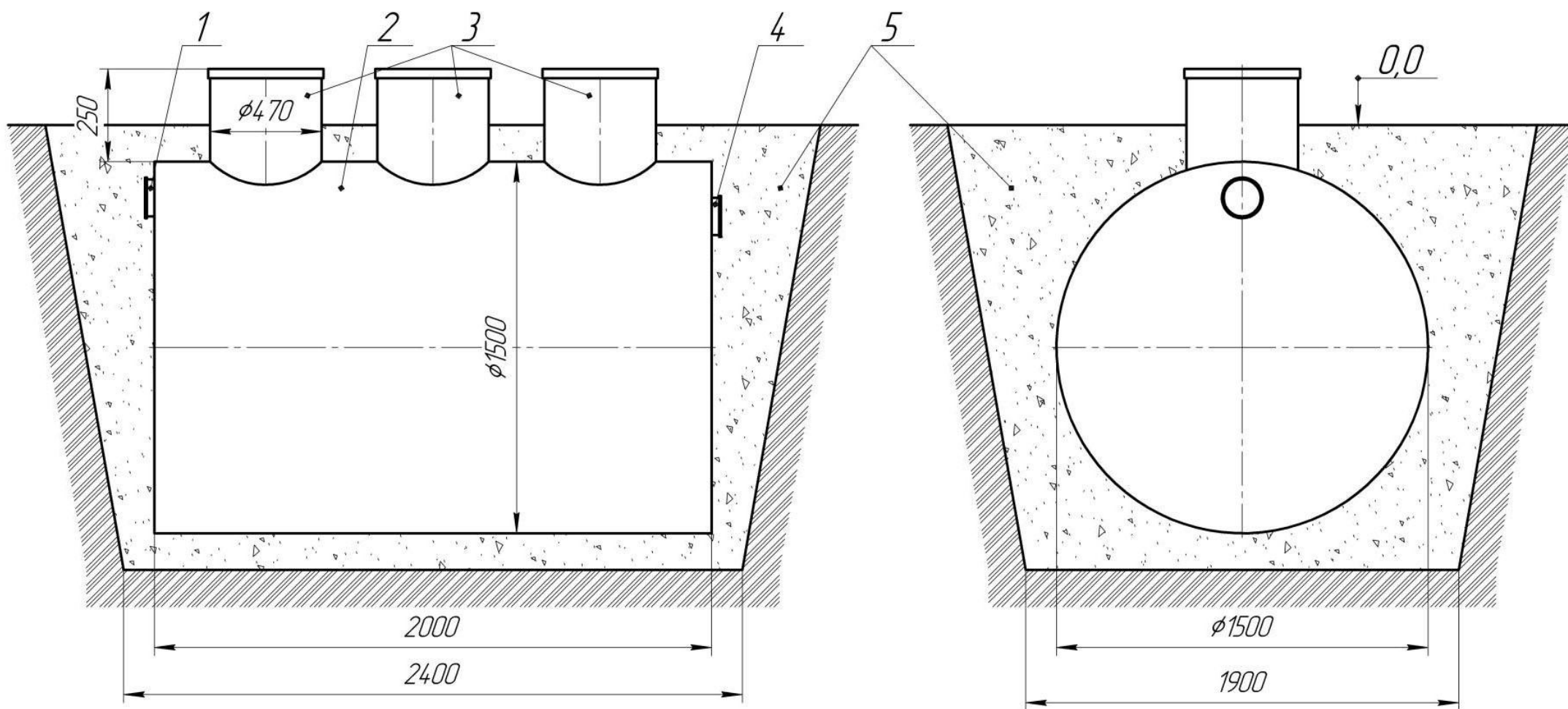
Рисунок А.1 Монтаж жироуловителя «Жирожор 25-1680» на подготовленное песчаное основание
