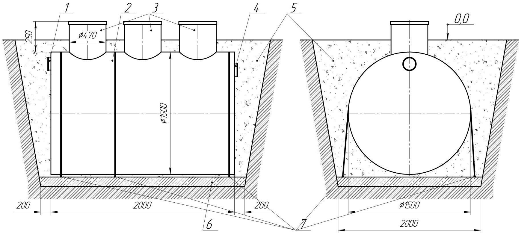
Рисунок А.1 Монтаж жироуловителя «Жирожор 25-1680» на ж/б основание
