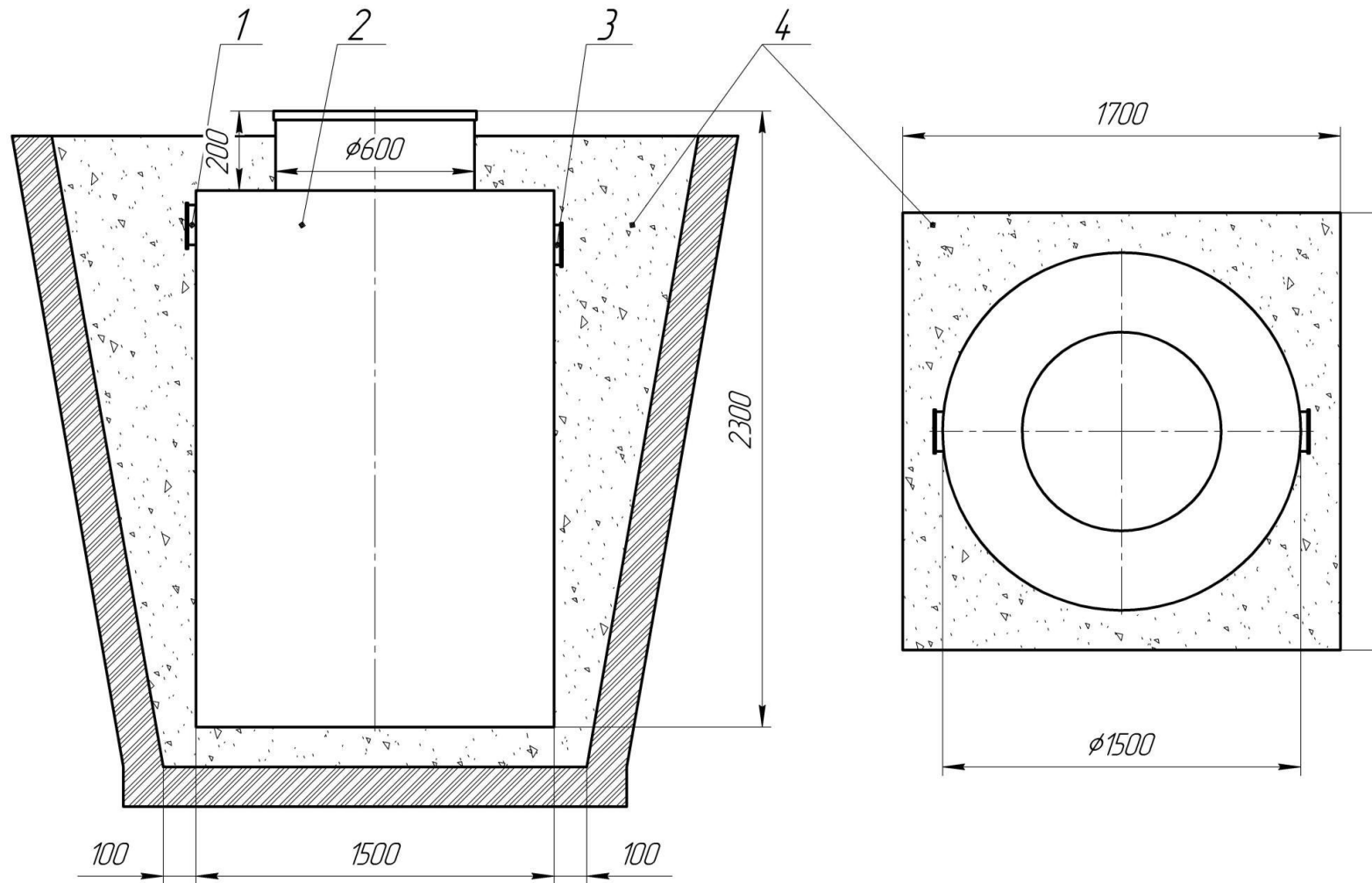
Рисунок А.1 Монтаж жирословителя «Жирословор 18-1000» на подготовленное песчаное основание
