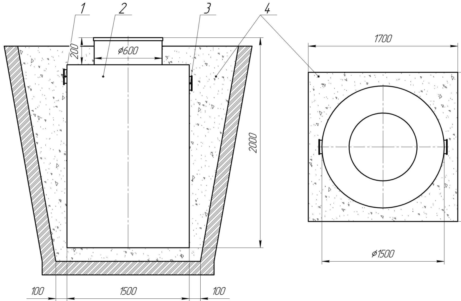
Рисунок А.1 Монтаж жирословителя «Жирословор 14-900» на подготовленное песчаное основание
