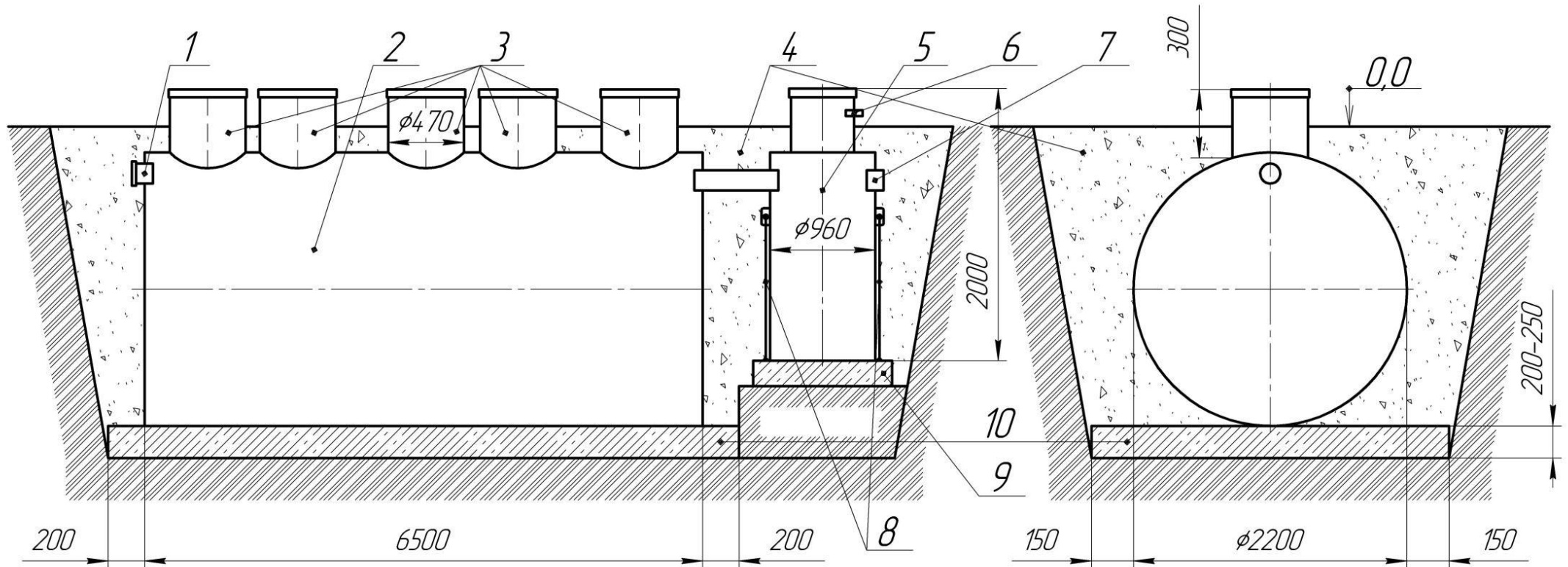
Рисунок А.6 Монтаж ЛОС «Биосфера 100 УФ» с ультрафиолетовым обеззаражителем сточных вод на ж/б основание
