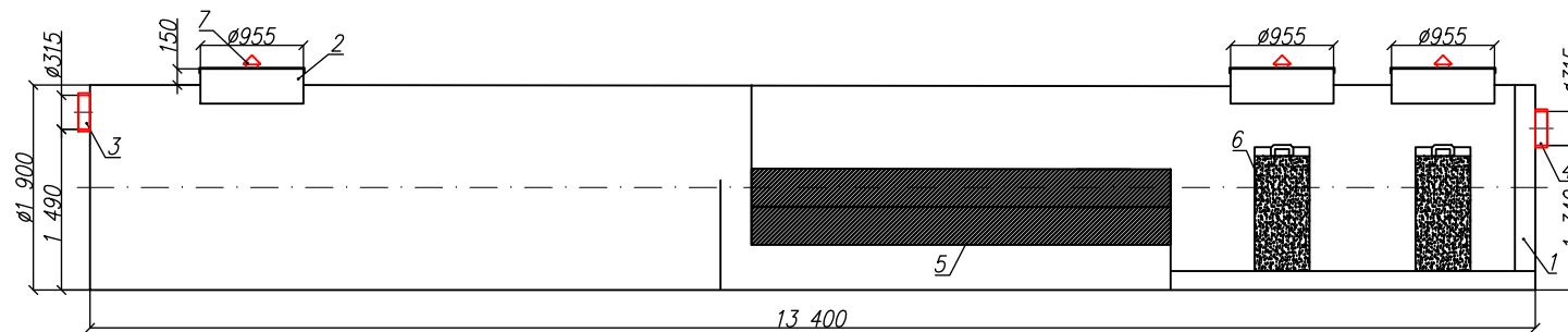
Разрез 1-1
