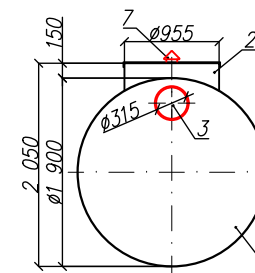
Вид спереди
