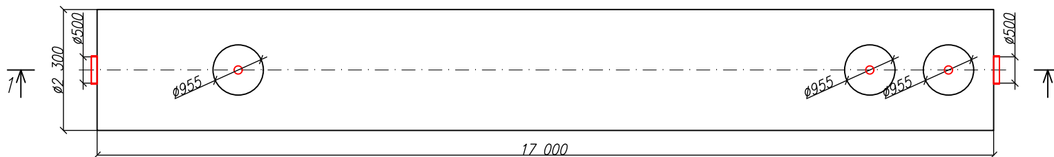
Вид сверху
